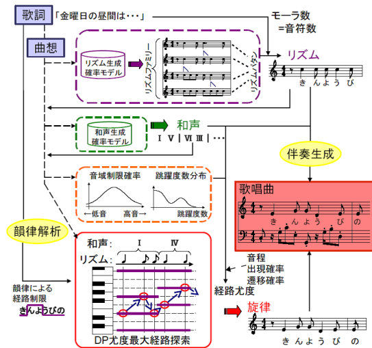
図 1 歌唱曲の作曲モデル
