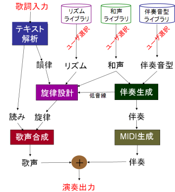
図 4 Orpheus のシステム構成
