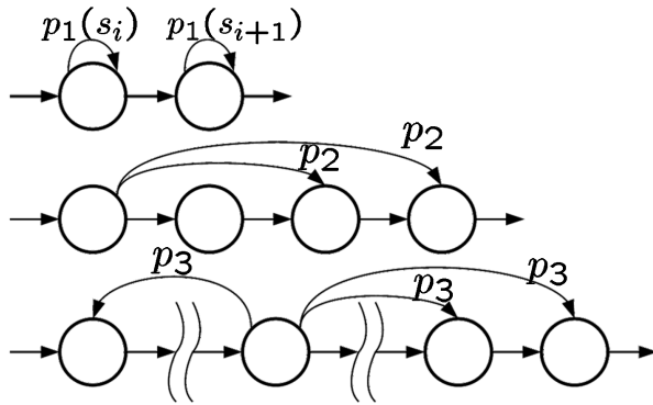
Fig. 2 遷移確率 p_1 , p_2 , p_3 を割り振った隠れマルコフモデル. p_1 : 音符 s_i の音長に対応. p_2 : 音符の脱落に対応. p_3 : 弾き飛ばし・弾き直しに対応.
